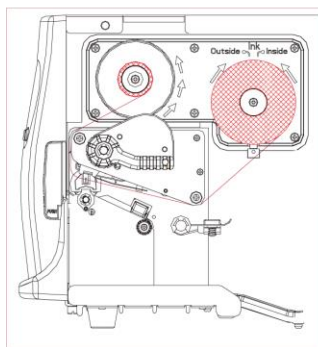
外卷式碳带安装方式 (即油墨面朝外)
