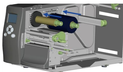
外卷式碳带安装方式 (即油墨面朝外)
