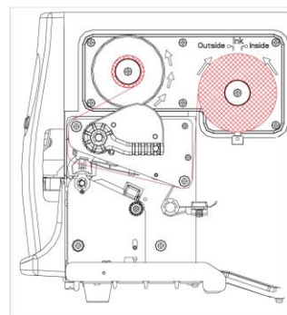
内卷式碳带安装方式 (即油墨面朝内)
